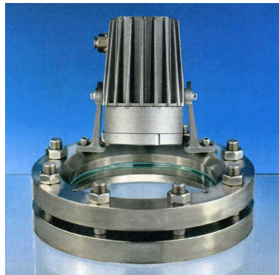
Caméra K07 Ex monté sur hublot DIN28120
