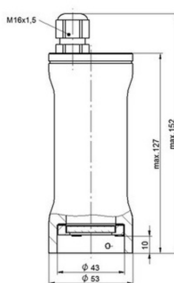
ESL 53LED-B pour montage à bride
